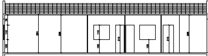
CORTE "BB" Esc.: 1/50
