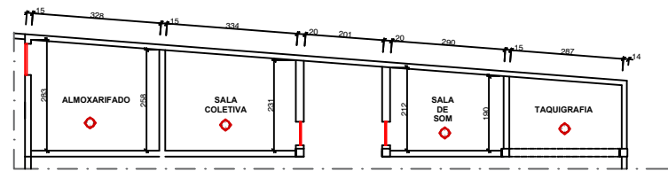
PLANTA BAIXA TÉRREO - SALAS ESC.: 1/50
