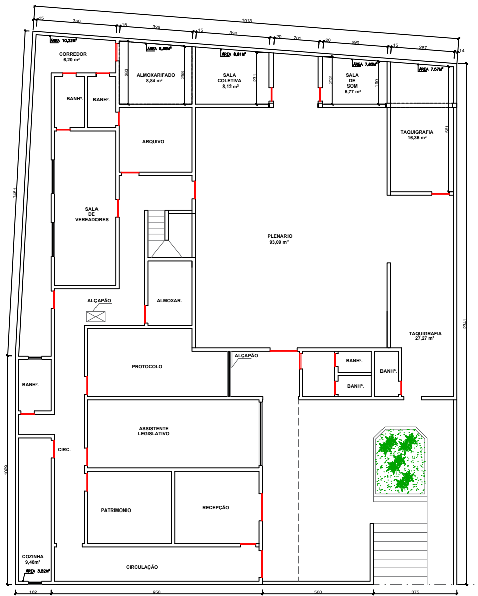
PLANTA BAIXA PAVT. TÉRREO ESTUDO DE ÁREA PARA REVESTIMENTOS ESC.: 1/80
