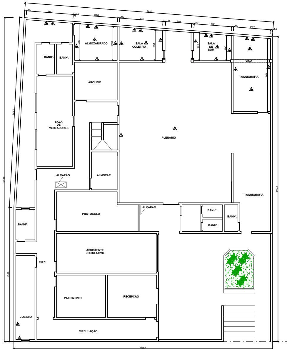
PLANTA BAIXA PAVT. TÉRREO ESTUDO DE COR/REVESTIMENTO Esc.: 1/50
